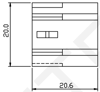
3x05 Pin
