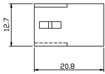
3x03 Pin
