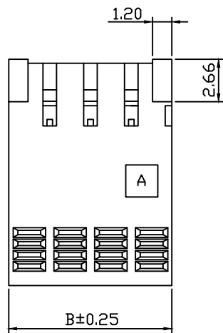
2x02P~2x07P
