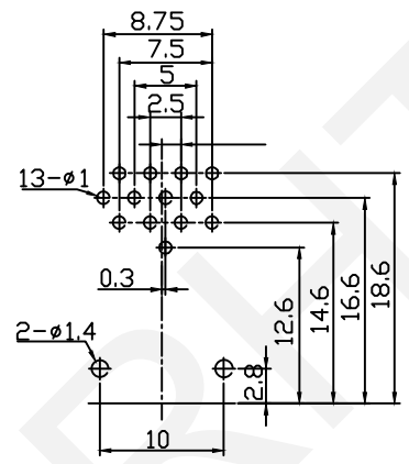
P.C.B LAYOUT
