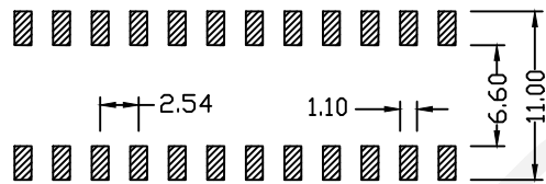
P.C.B. LAYOUT
