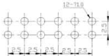
P.C.B HOLE DETAIL
